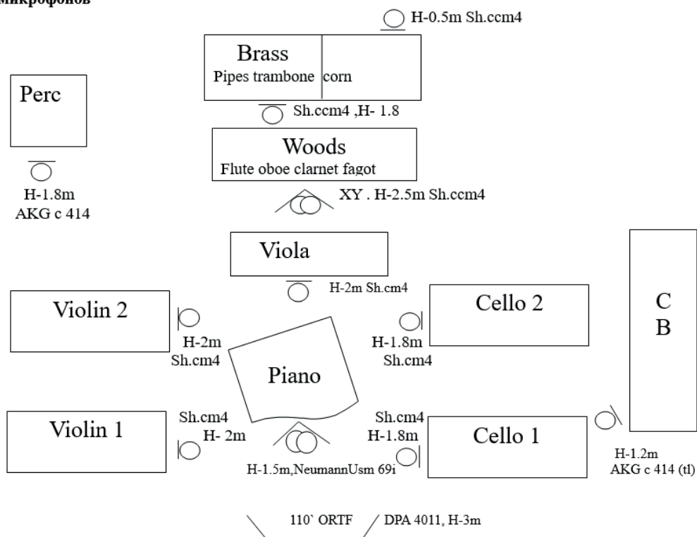
Схема – 1. Расстановка микрофонов
