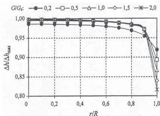
Рис. 2. Профили относительного уплотнения коллектора радиусом R = 3000 м, h = 50 м [2]
